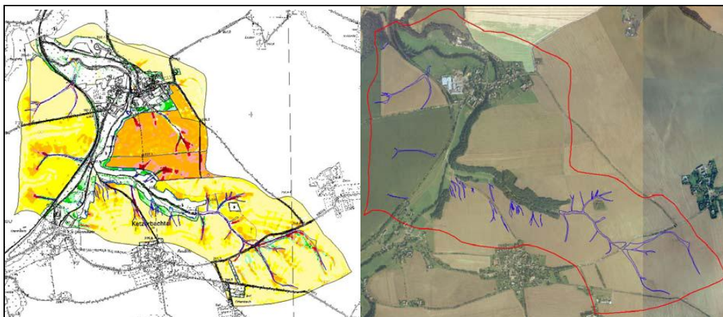
Abbildung 7: Erosionsrinnen und Bodenabtrag für Beispielgebiet 2 (Schob und Schmidt 2006)
