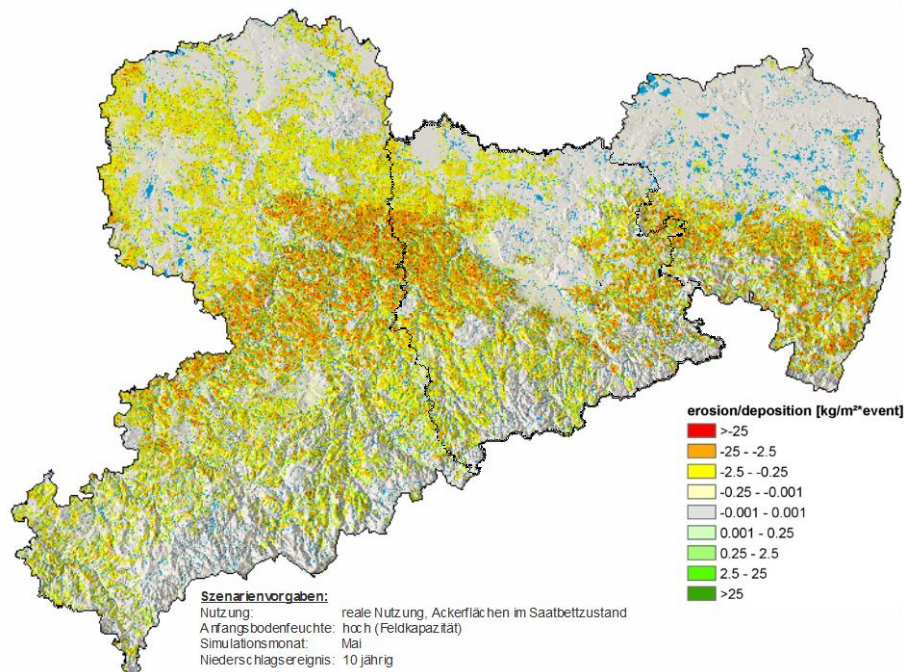
Abbildung 1: Erosionsgefährdung berechnet mit EROSION 3D für ein 10-jähriges Niederschlagsereignis (Schindewolf 2010)
