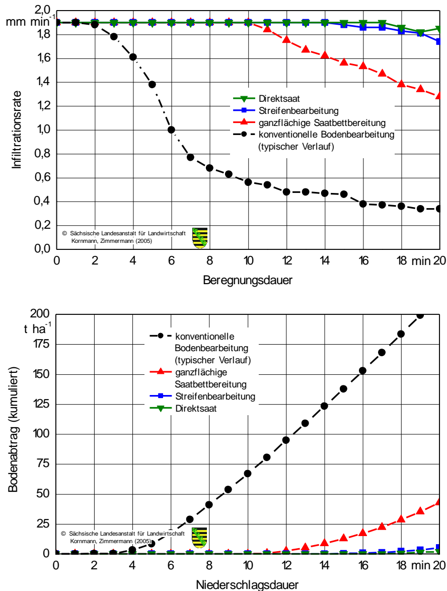
Abbildung 9: Auswirkungen unterschiedlicher Bodenbearbeitung zu Mais auf die Wasserinfiltration (oben) und den Bodenabtrag (unten) in einem Regensimulationsversuch, Körnermais, 38 mm/20 min (Schmidt 2010)
