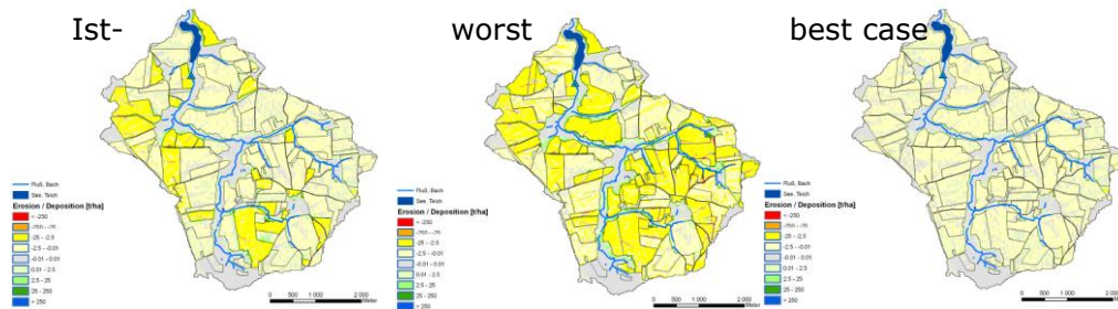
Abbildung 6: Erosion für das Gebiet und drei Szenarien (Kornmann et al. 2008)
