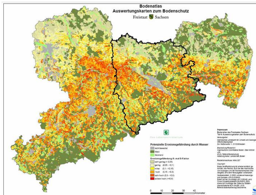
Abbildung 2: Potenzielle Erosionsgefährdung durch Wasser nach ABAG (Bodenatlas Sachsen 2008)
