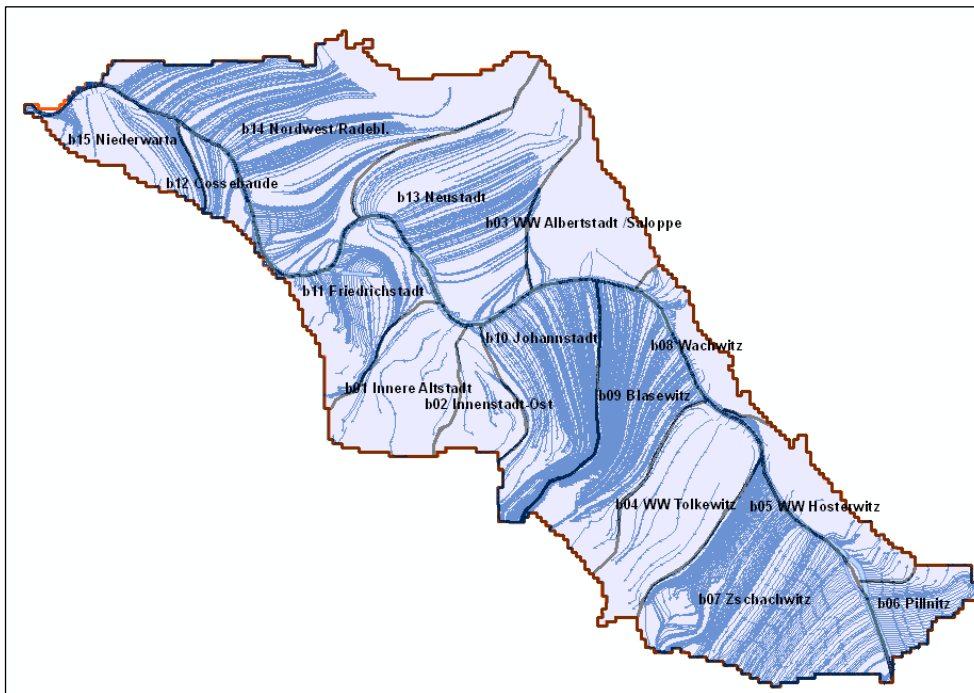
Abbildung 10: Bilanzgebiete im pleistozänen Elbtalgrundwasserleiter Dresdens
