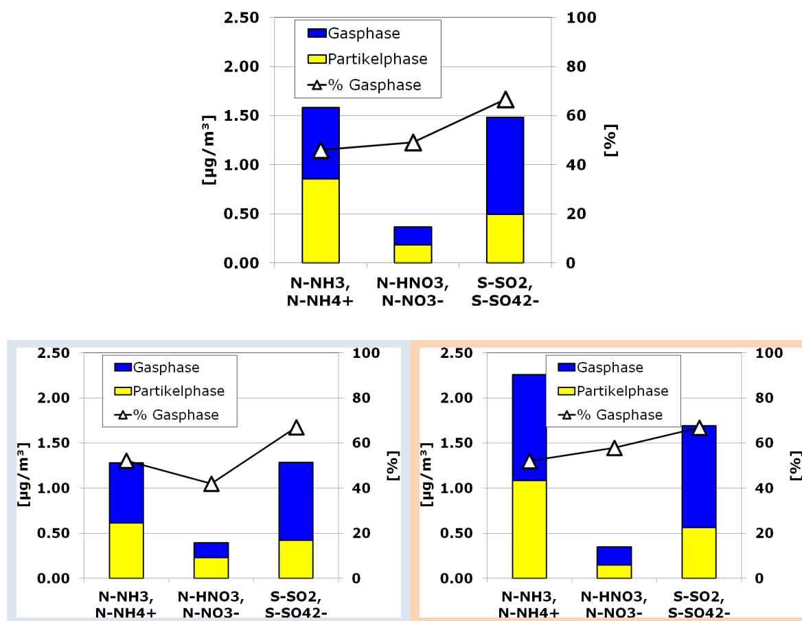
Abbildung 19: Mittlere Luftkonzentrationen von NH 3 , HNO 3 , SO 2 im Vergleich zu NH 4 + , NO 3 - , SO 4 2- in der korrespondierenden Partikelphase für die Ankerstationen Oberbärenburg. blau : für vorherrschende Windrichtungen aus West, orange : für vorherrschende Windrichtung aus Ost
