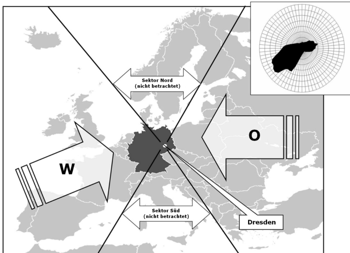
Abbildung 8: Lage von Dresden in Europa. und die beiden betrachteten großräumigen Anströmungen West (W) und Ost (O).. Es sind die Anströmungssektoren West (W, maritime und kontinentale Luftmassen) und Ost (O, kontinentale Luftmassen) gekennzeichnet. Zum Vergleich ist die Windrose der Messstation Melpitz gezeigt.
