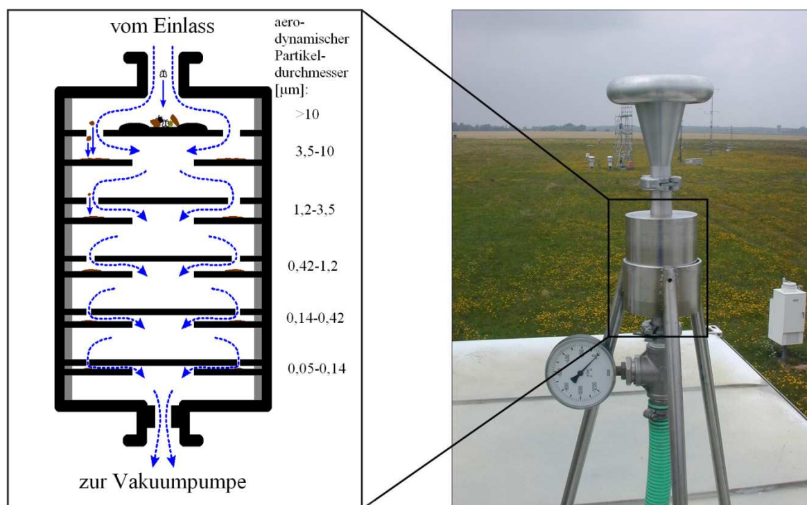
Abbildung 3: Fünfstufiger BERNER-Niederdruckimpaktor (Querschnitt und Ansicht mit anisokinetischem Einlasskopf).
