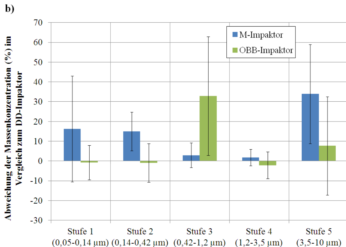
Abbildung 7: Vergleichsmessung der drei verwendeten Impaktoren am TROPOS. a) gesammelte PM 10 -Massenkonzentrationen in den drei Läufen. b) Abweichung der gesammelten PM 10 -Massenkonzentration der Impaktoren aus M und OBB im Vergleich zu derjenigen des DD-Impaktors. Die Fehlerbalken geben die Standardabweichung dieser Abweichung wieder (Mittel über drei Läufe).
