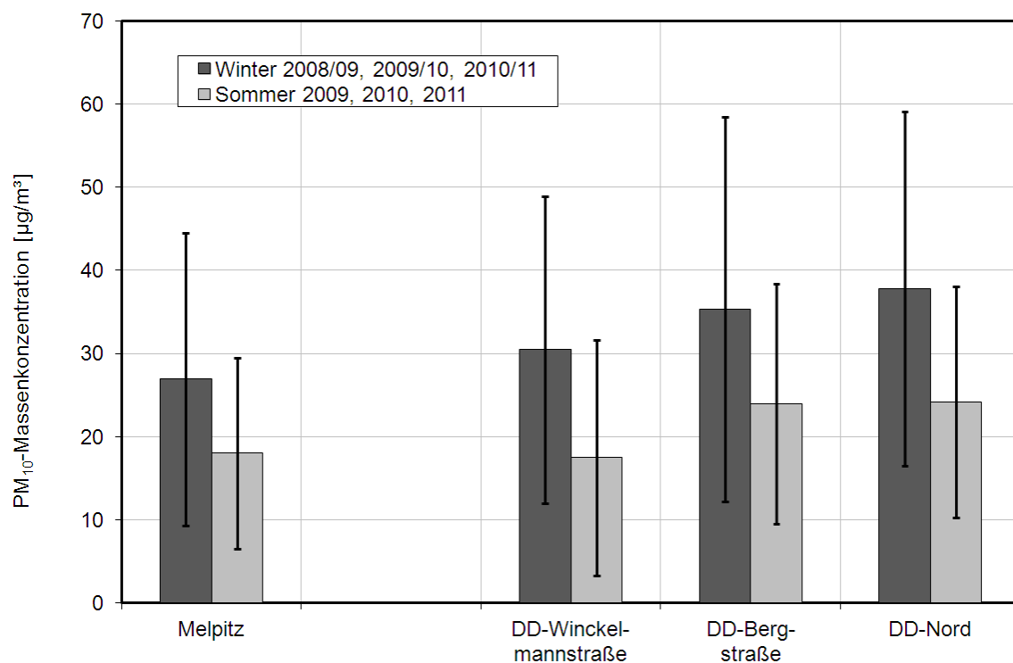
Abbildung 5: Vergleich des Verlaufes der PM 10 -Konzentrationen für drei Stationen in Dresden und für Melpitz (oben) und Vergleich des Dreijahresmittelwertes (unten). Die eingezeichnete Standardabweichung ist hier ein Maß für die Variabilität der täglichen PM 10 -Messungen (Zeitraum: September 2008 bis August 2011).
