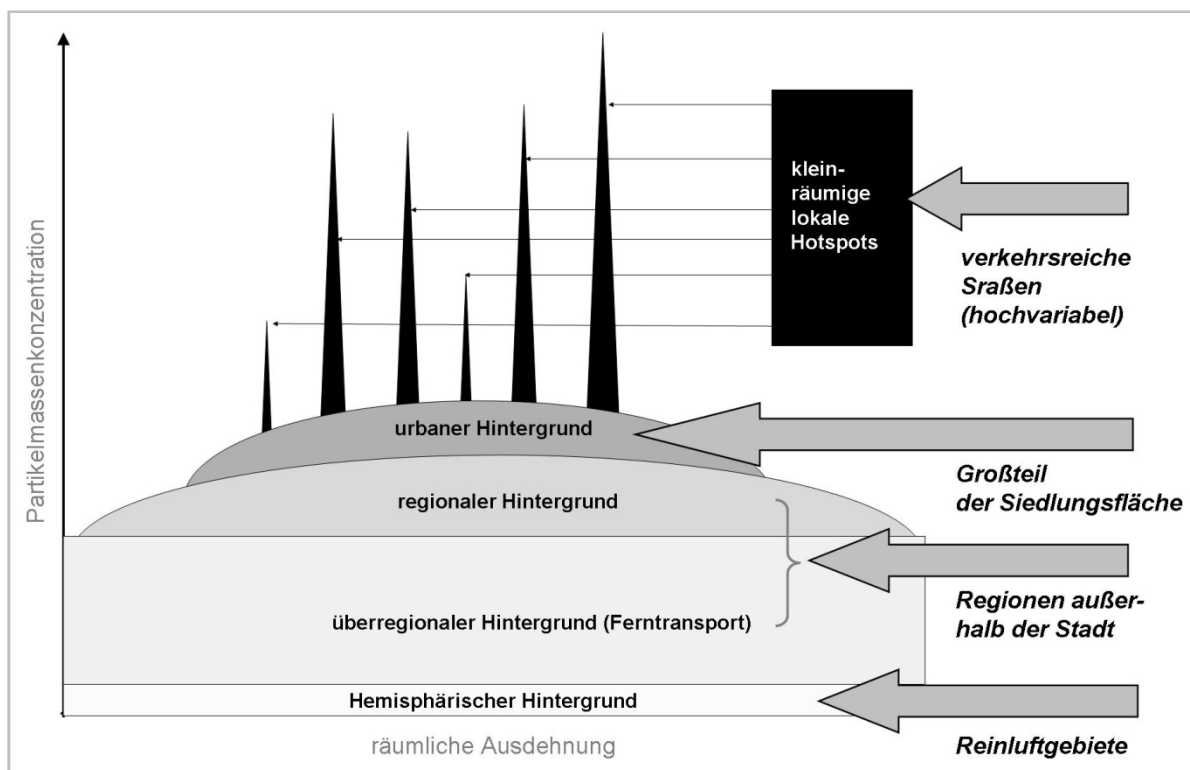
Abbildung 1: Schematische Darstellung der Beiträge zur Partikelmassenkonzentration in einer Stadtregion (in Anlehnung an Lenschow et al., 2001).
