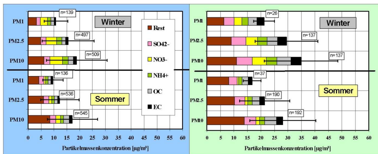
Abbildung 2: Mittelwerte für PM_1 -, PM_{2.5} - und PM_{10} -Konzentrationen für die wasserlöslichen Hauptionen, den nicht analysierten „Rest“ und organischen (OC) sowie elementaren (EC) Kohlenstoff für fünf Sommerhalbjahre (2004-2008) und fünf Winterhalbjahre (05/2004-09/2008), unterschieden nach großräumiger Anströmung: WEST blauer Rahmen, OST grüner Rahmen. Die angegebenen Fehlerbalken sind die Standardabweichungen für die Partikelmassenkonzentration und zeigen die Variabilität der Tagesmittelwerte. PM_1 wurde jeden 6. Tag gemessen. n ist die Anzahl der gemittelten Tagesmittelkonzentrationen.
